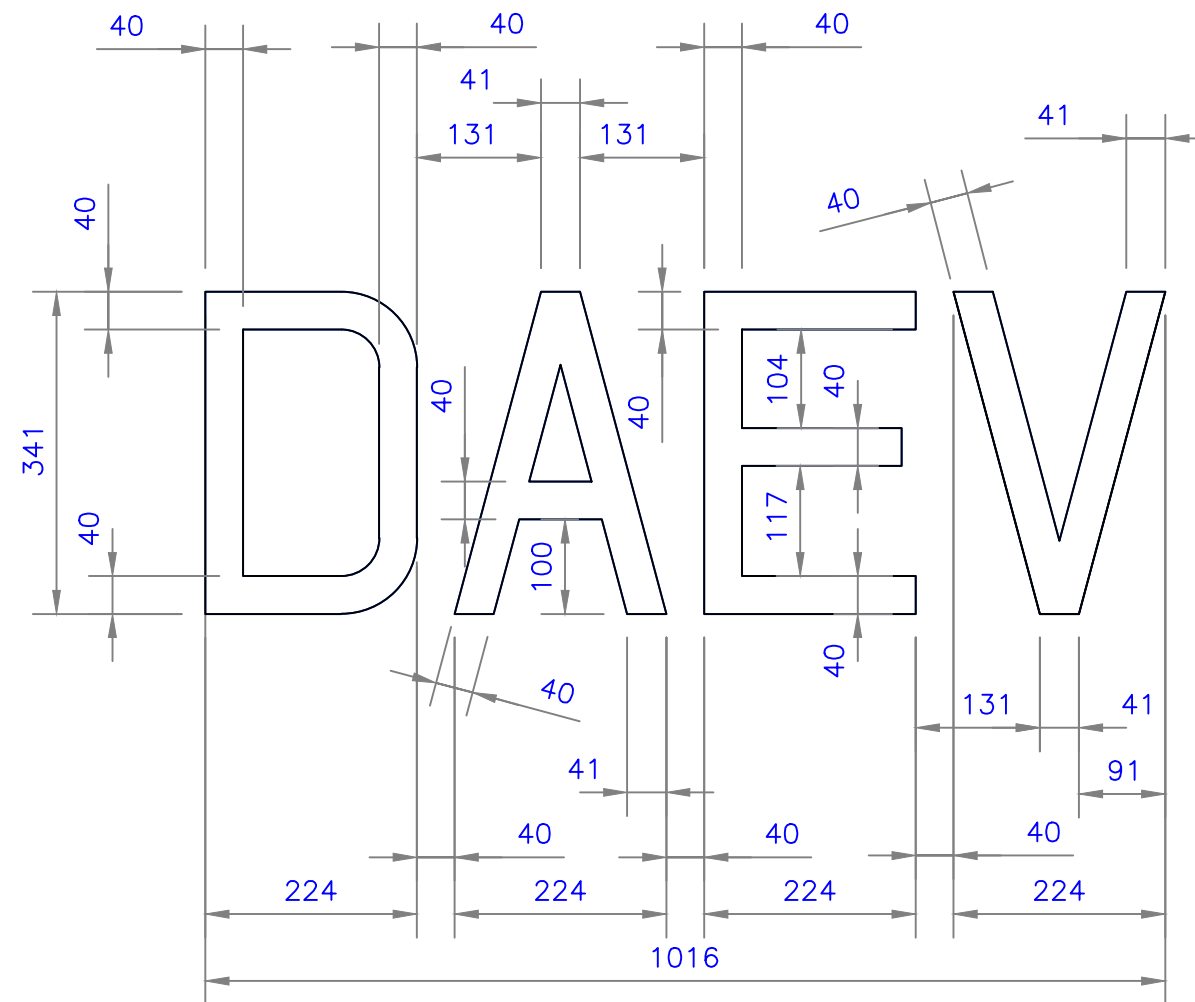
LOGOTIPO P/ TANQUE DE 30m 3 Esc. 1:8
